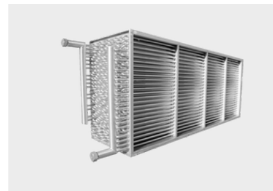
Récupérateurs de chaleur industriels sur fumée
